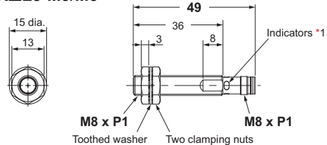
E2E-X□L8-M1
