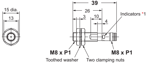
E2E-X□8-M1
