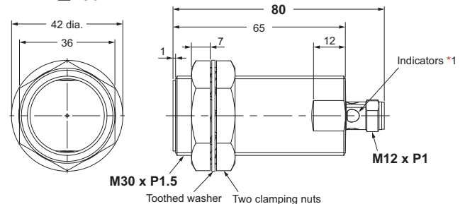
E2E-X□L30-M1
