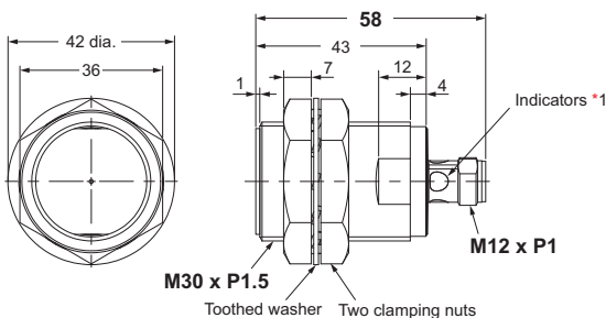
E2E-X□30-M1
