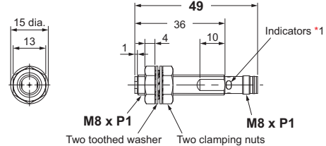
E2E-X□L8-M1
