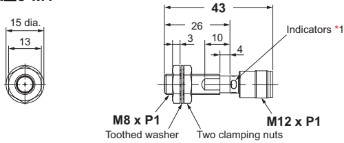
E2E-X□12-M1
